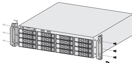
图2-1 角铁安装示意图
