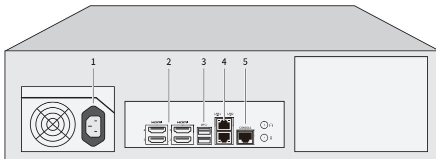
图1-3 TL-TUMS3500-AI后面板编码示意图
